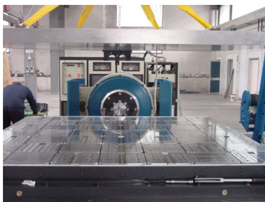
Il laboratorio per lo studio degli effetti delle radiazioni sui materiali per lo spazio presso il Polo scientifico e didattico di Terni The Laboratory for the study of radiation effects on materials for outer space at the Research and Didactic Center in Terni
